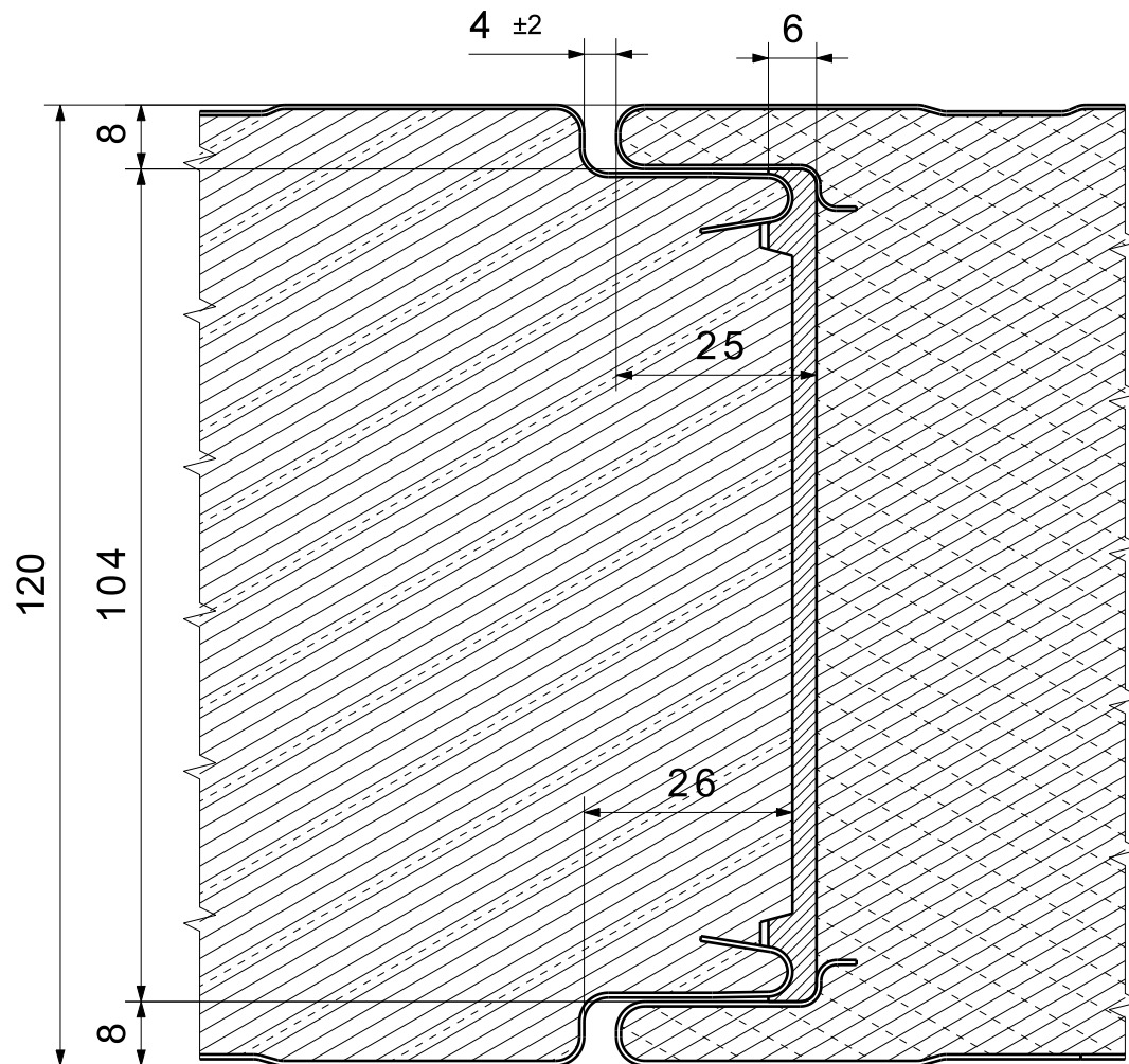
Vorderansicht Maßstab: 1:1
