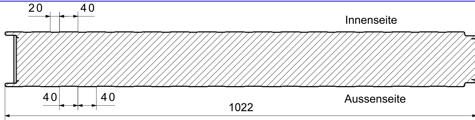
Vorderansicht Maßstab: 1:5
