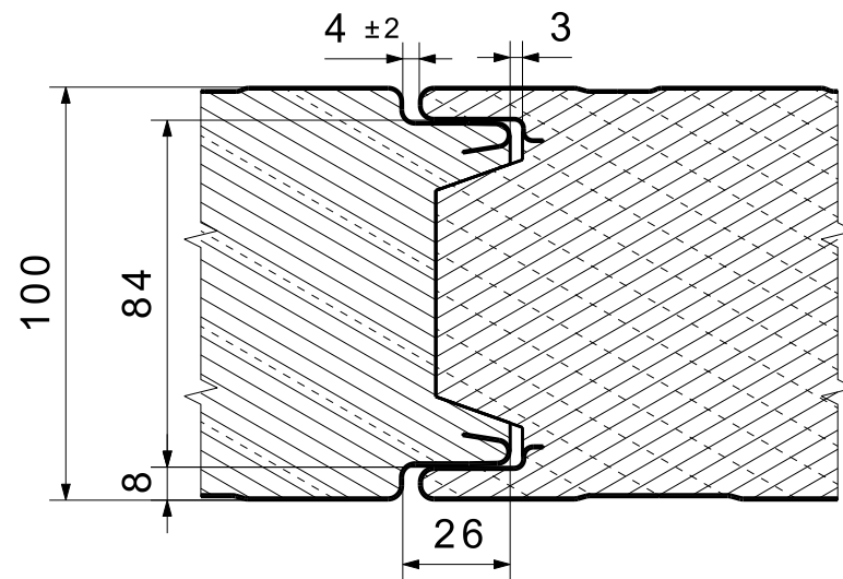
Vorderansicht Maßstab: 1:2
