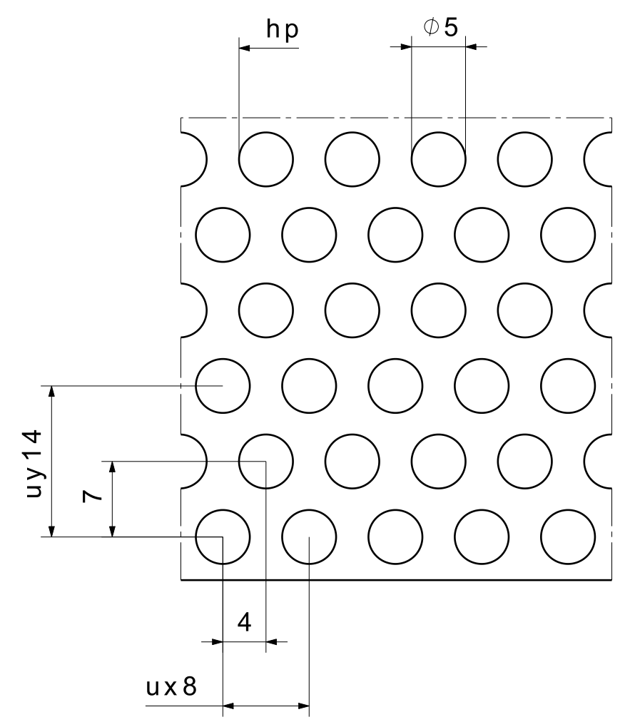
Detail C Maßstab: 2:1
