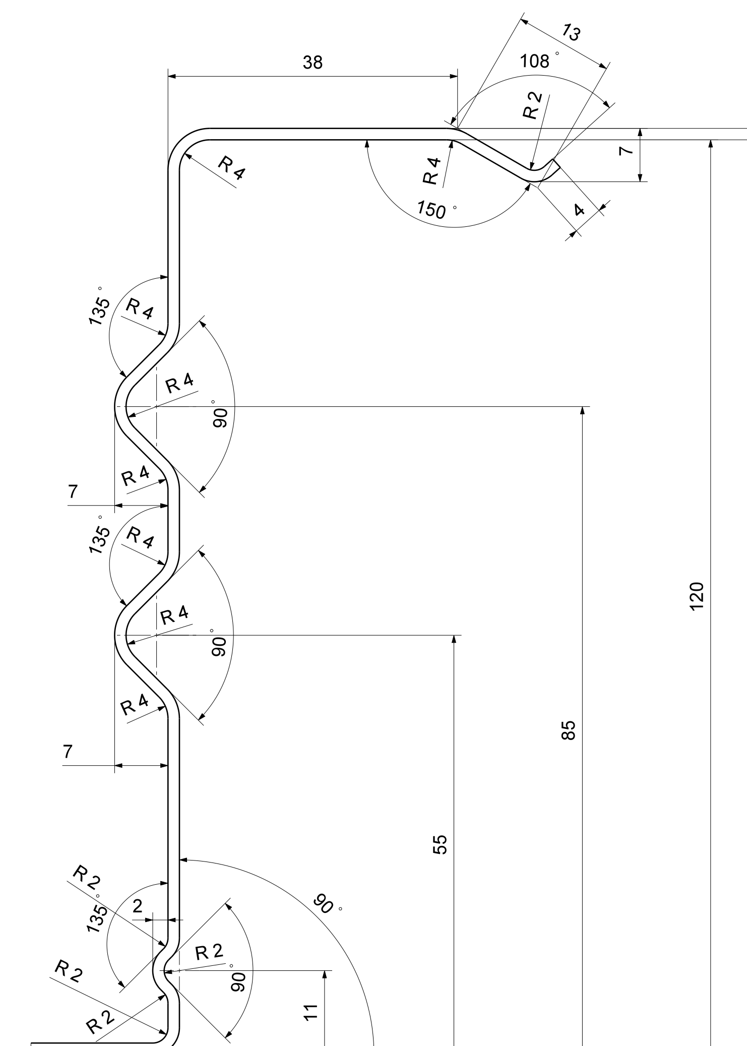
Detail A Maßstab: 2:1
