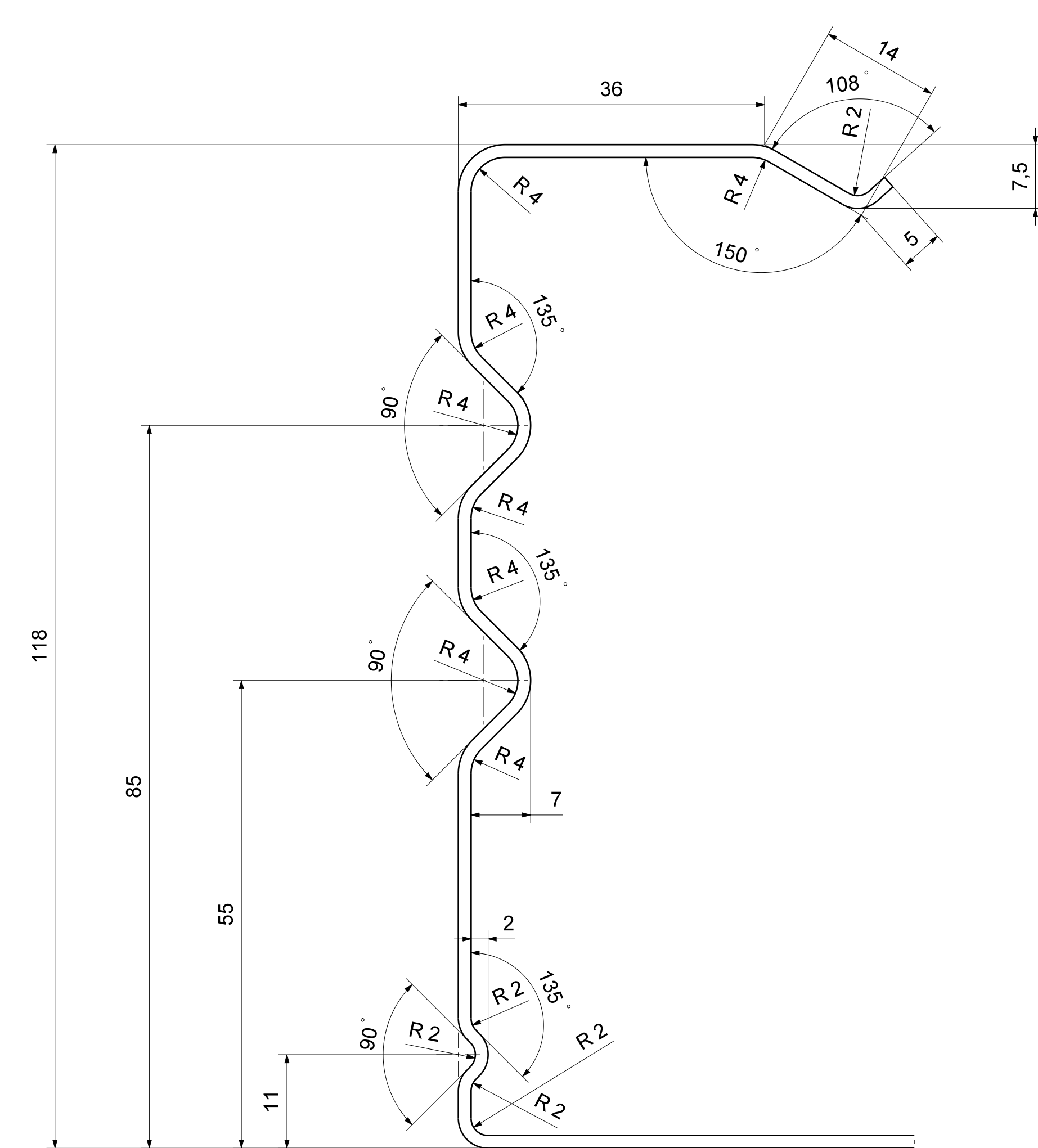
Detail B Maßstab: 2:1
