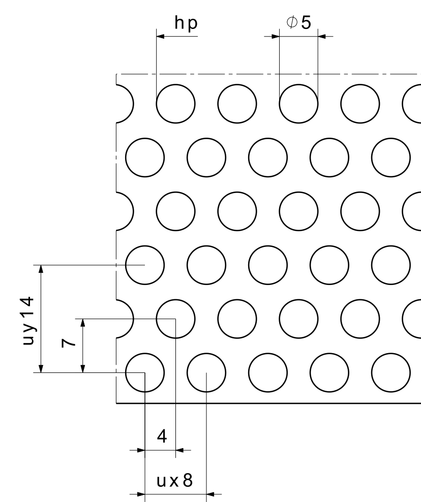
Detail C Maßstab: 2:1
